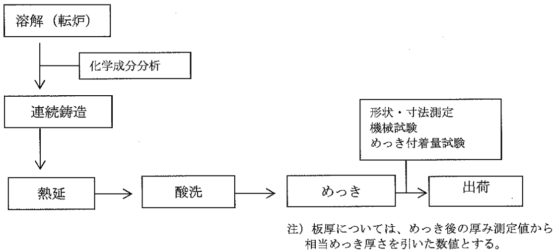
図1 製造工程及び検査工程
