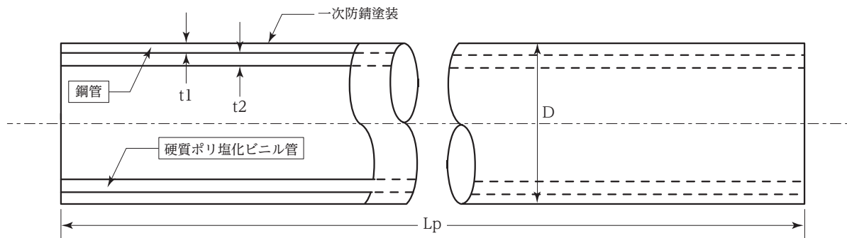
備考1. 鋼管の寸法許容差 (mm)
