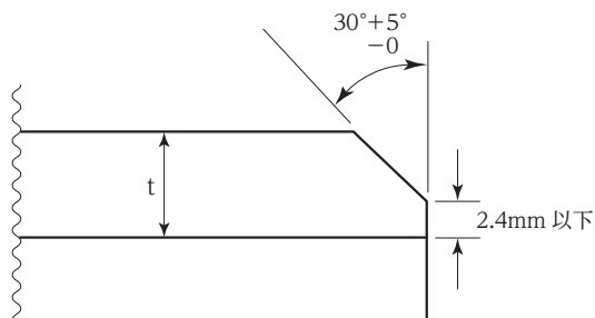
(B) 部 詳 細 図
