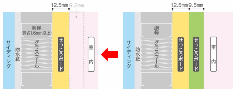
一般的な防火構造
