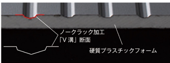
スターラインプライム®-HJの防火構造
