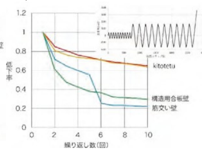
■1/30radの変形を繰り返し与えた実験データ
