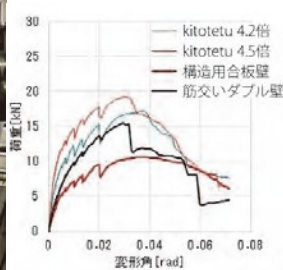
■荷重変位曲線
