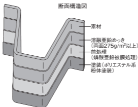
■塗装構造図
