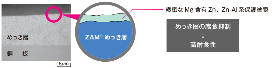
塩水噴霧試験後(4時間)にめっき層表面に形成する保護被膜 (板厚：0.8mm、めっき付着量：90/90 g/m 2 、無処理)
