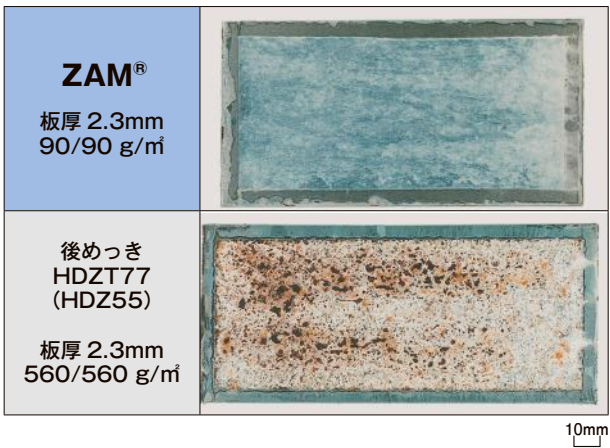
二酸化硫黄試験 450時間後の外観写真
