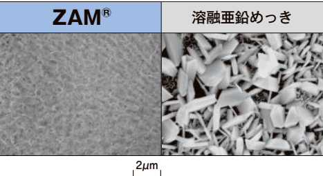
塩水噴霧試験後(4時間)にめっき層表面に形成する保護被膜 (板厚：0.8mm、めっき付着量：90/90 g/m 2 、無処理)
