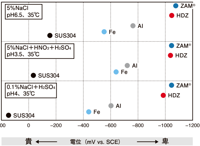
浸漬電位測定水溶液
