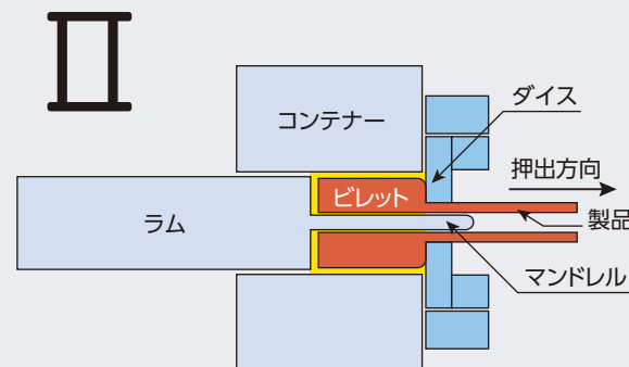
中空形鋼の押出
