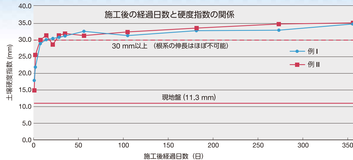
図3：施工後の硬化確認試験結果例（山中式土壌硬度計による当社調査）
