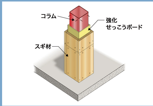
木質耐火技術 (木鉄ハイブリッド耐火柱) (BCJ評定-STO311-01)
