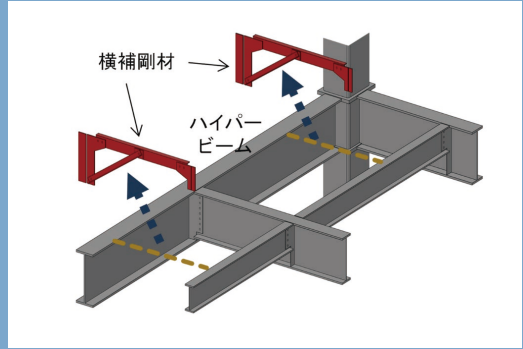
横補剛材省略工法
