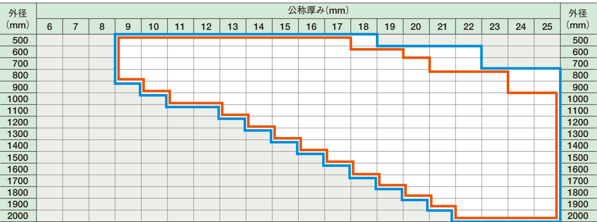
鋼管矢板 製造範囲 400N/mm 2 鋼・490N/mm 2 鋼
