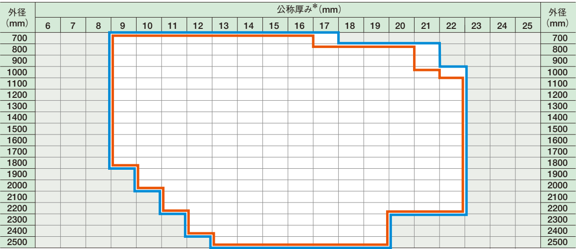
外面・内面突起付鋼管杭 製造範囲 400N/mm 2 鋼・490N/mm 2 鋼
