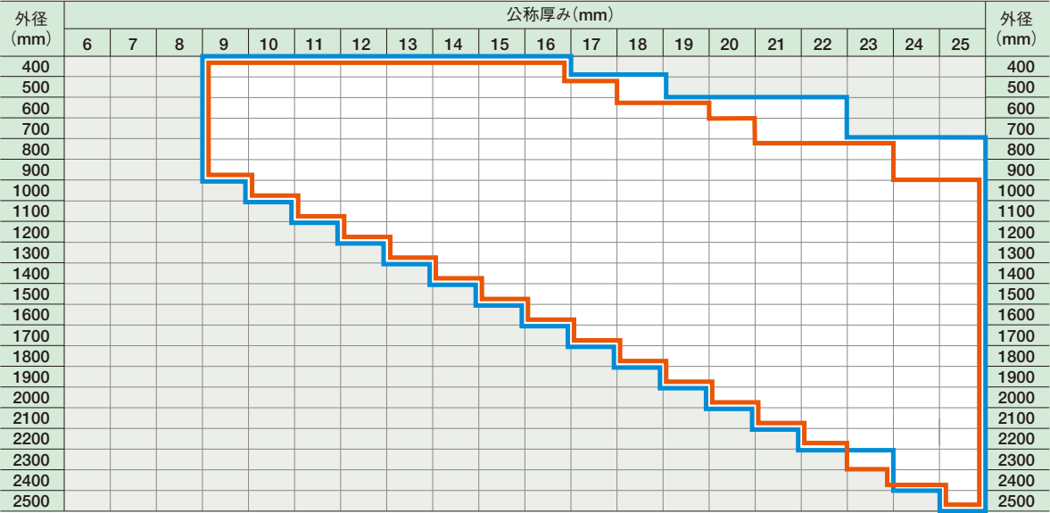
鋼管杭 製造範囲 400N/mm 2 鋼・490N/mm 2 鋼
