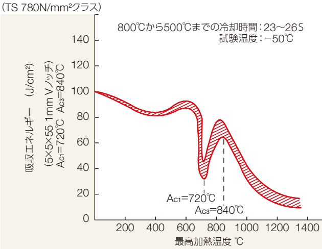
図8. 高張力鋼熱影響部の脆化領域
