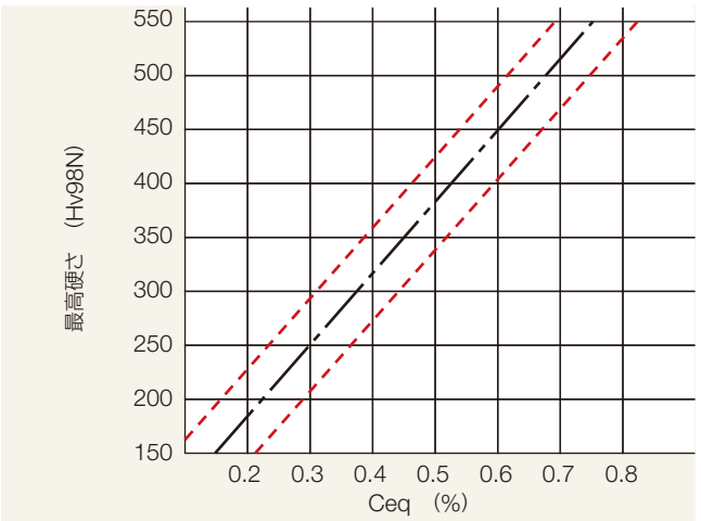
図7. 最高硬さと炭素当量
