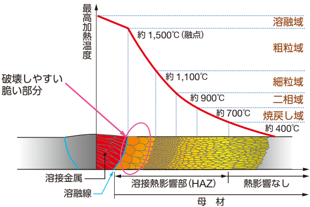
図5. 鉄－炭素系平衡態図と溶接熱サイクルとの関係
