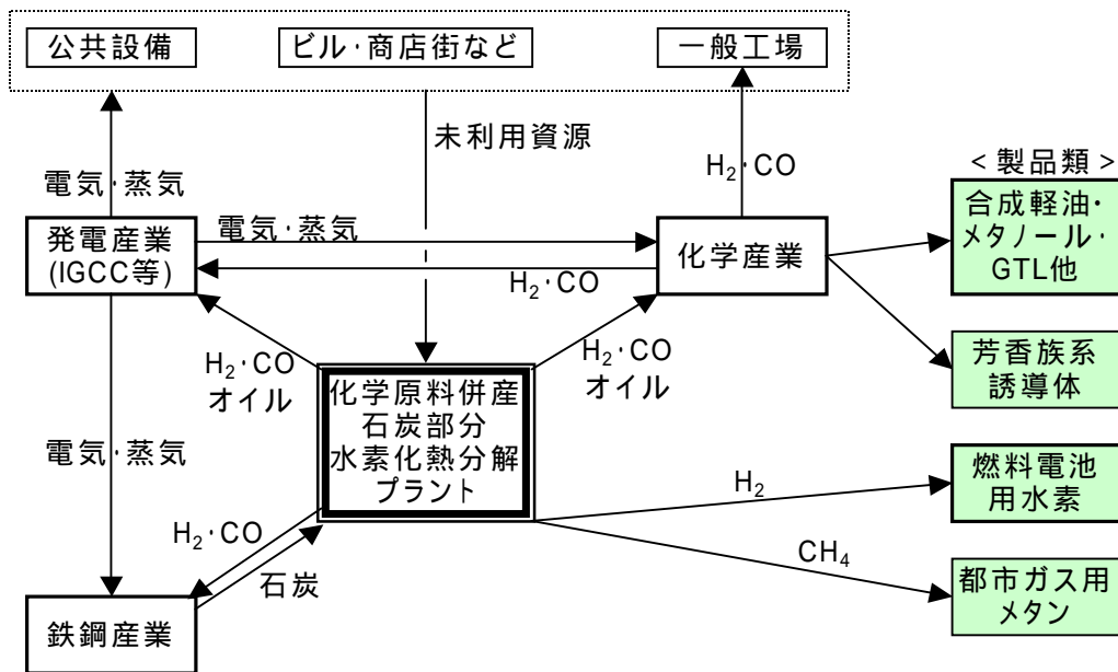
図2 エネルギー / 物質供給の業界融合型複合事業の概念
