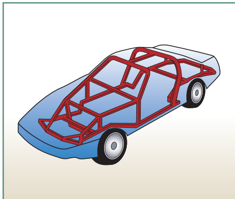
スペースフレームボディ構造
