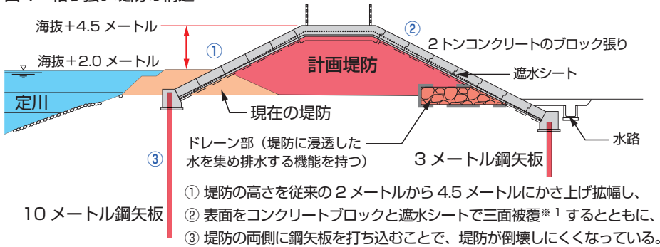
図1 粘り強い堤防の構造
