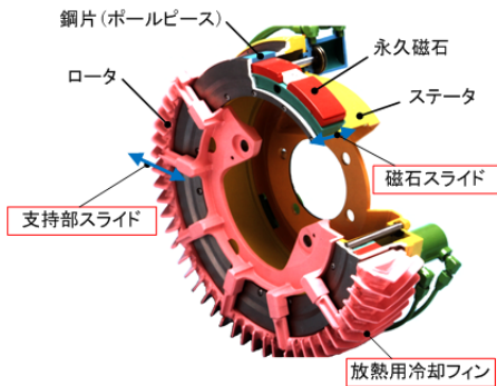
図3 初期型 外観
