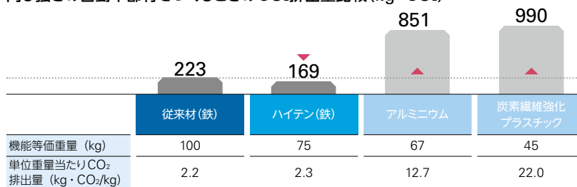
同じ強さの自動車部材をつくる時のCO 2 排出量比較(kg・CO 2 )
